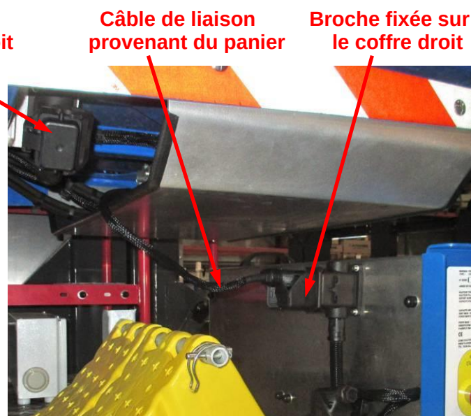
Câble « panier » connecté à la broche située sur le coffre = Recharge de la batterie lithium
