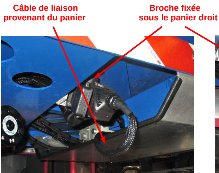
Câble « panier » connecté à la broche située sous le panier = Utilisation de la batterie en mode travail
